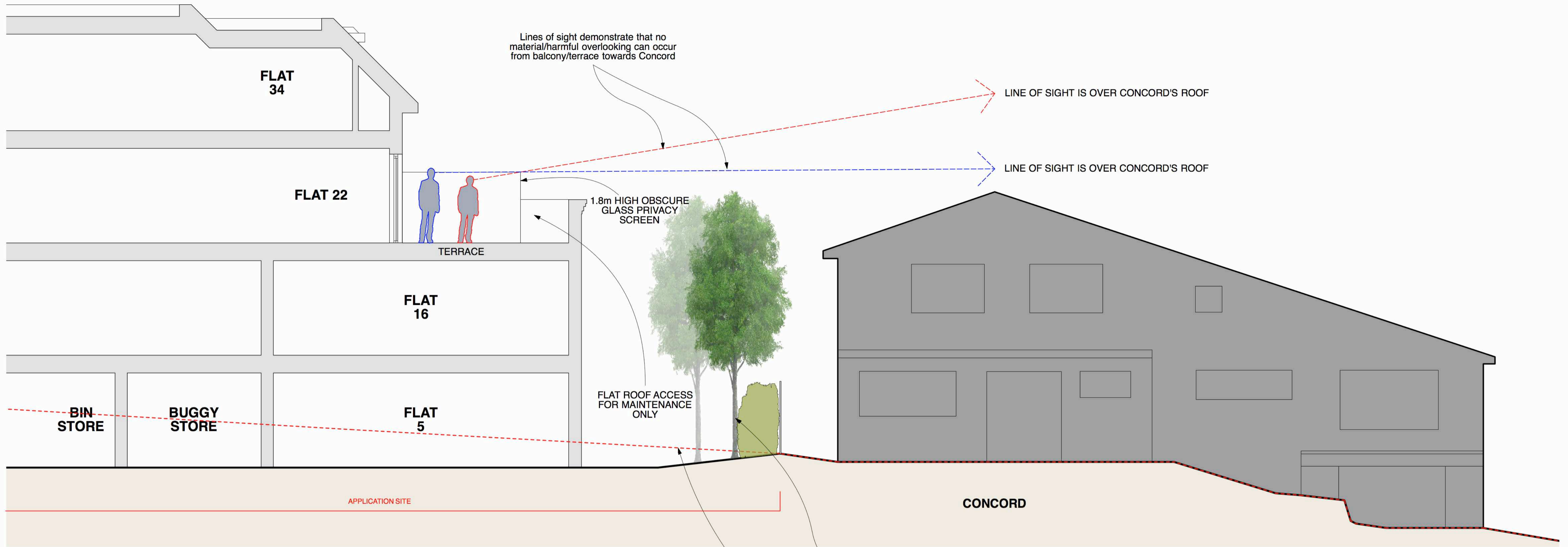
Section A-A Scale 1:50 @ A1 / 1:100 @ A3
